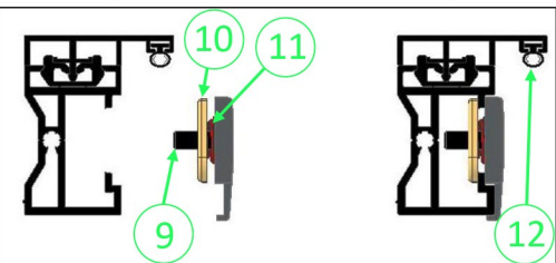
Vue de dessus: Gâche de fermeture
