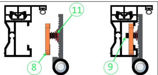
Vue de dessus: Paumelle inférieure
